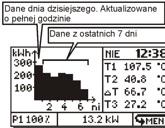
Uzysk ciepła w oknie głównym.
